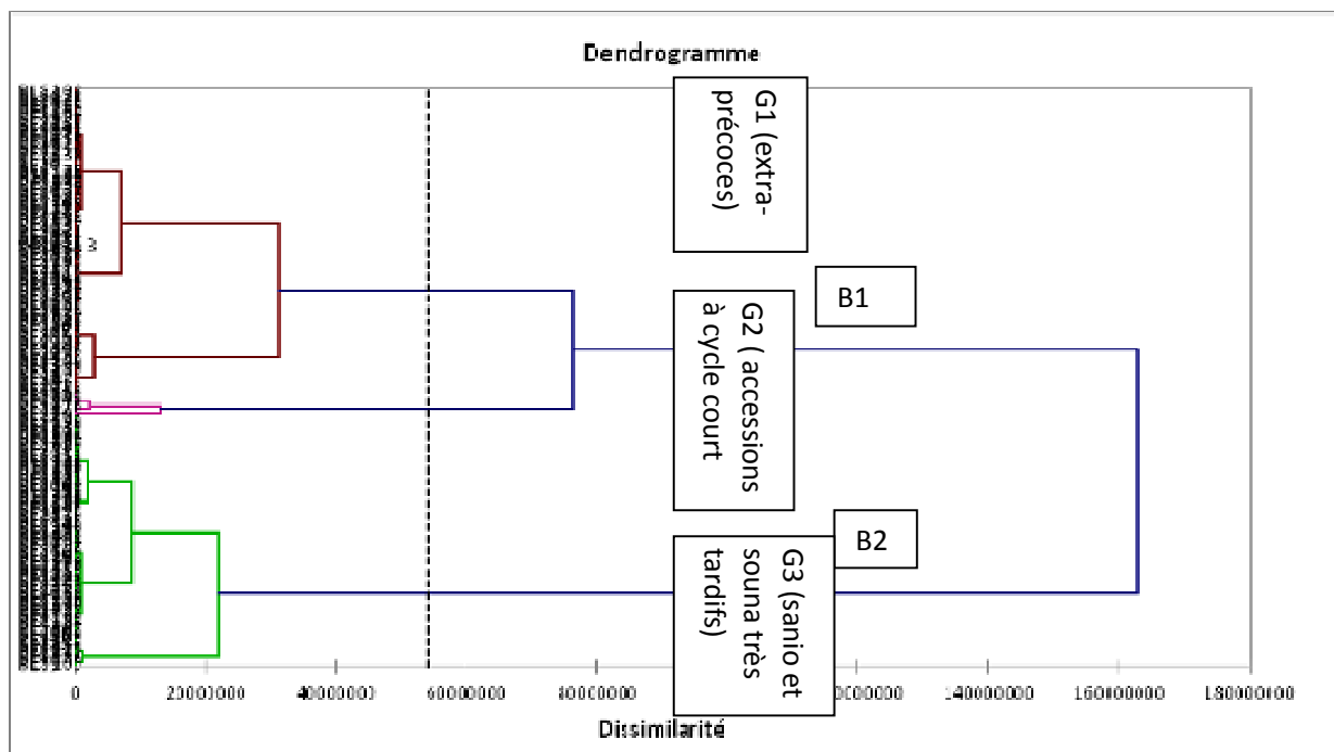
Figure 5 : Présentation phylogénétique des accessions de la collection nationale de mils locaux du Sénégal.
