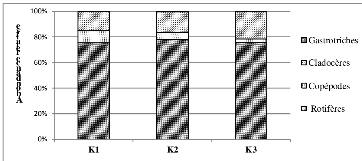
Figure 1 : Contribution des rotifères, des copépodes, des cladocères et des gastrotriches à l'abondance du zooplancton au niveau de chaque station.
