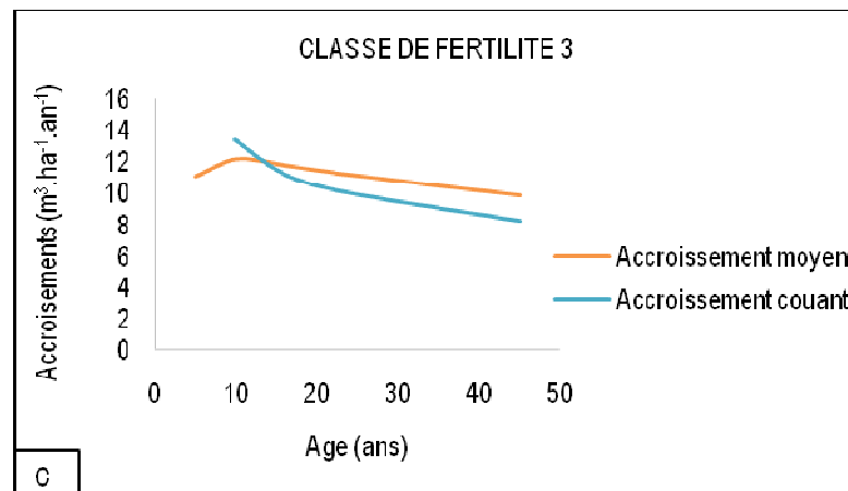
Figures 5 : Accroissements moyens et courants en fonction des classes de fertilité 3 et 4 du sol (avec C-Graphes des classes de fertilité 3 ; D-Graphes des classes de fertilité 4)
