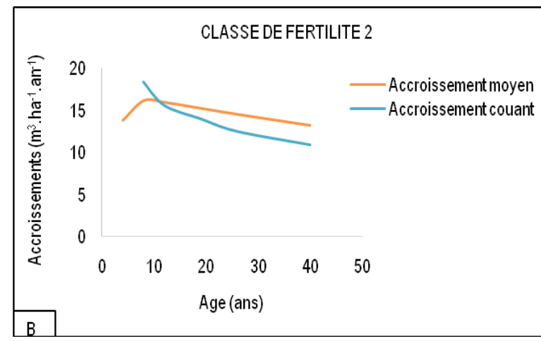
Figures 4 : Accroissements moyens et courants en fonction des classes de fertilité 1 et 2 du sol (avec A-Graphes des classes de fertilité 1 ; B-Graphes des classes de fertilité 2)
