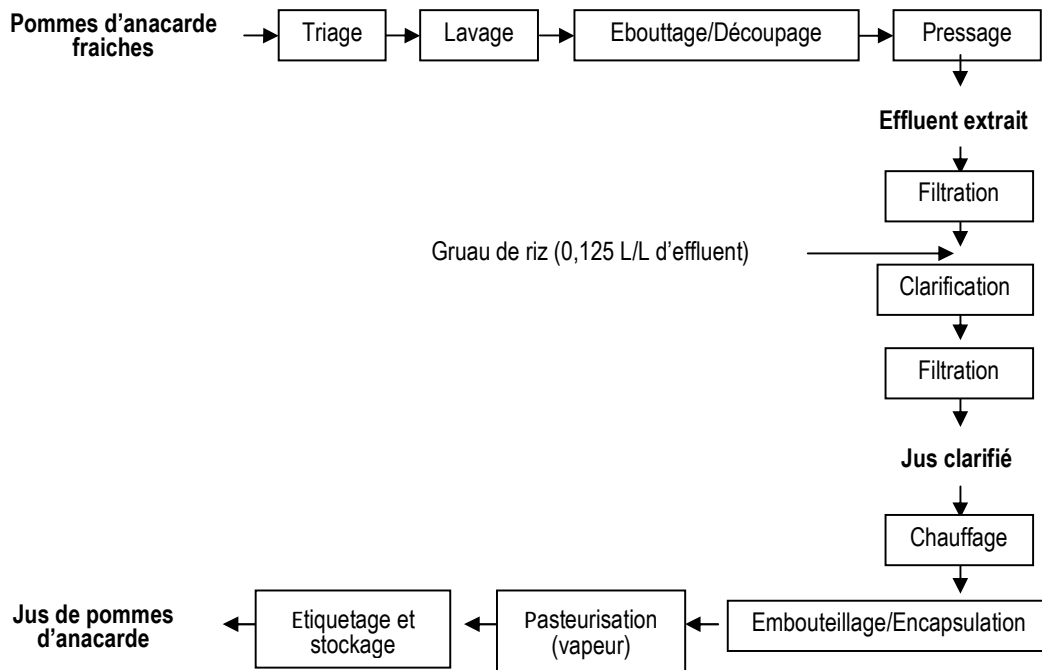
Figure 1 : Diagramme technologique de la production du jus de pommes d'anacarde.
