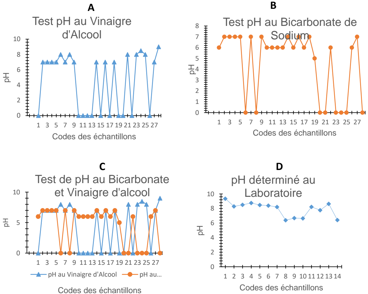
Fig. 3. Diagramme illustrant les tests réalisés sur le terrain et les analyses effectuées au laboratoire (A=test au vinaigre d’alcool, B=test au bicarbonate de sodium, C=test au vinaigre blanc et au bicarbonate de sodium, D=pH déterminé au laboratoire
